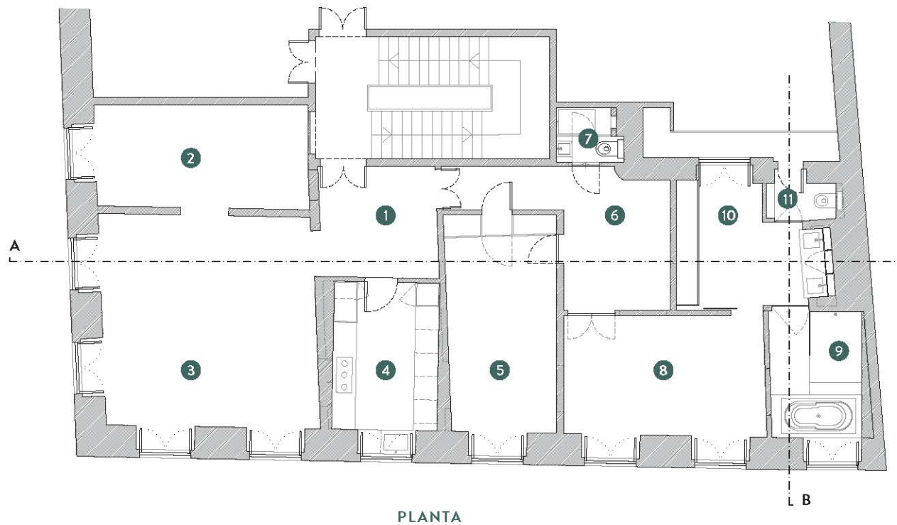
PLANTA
